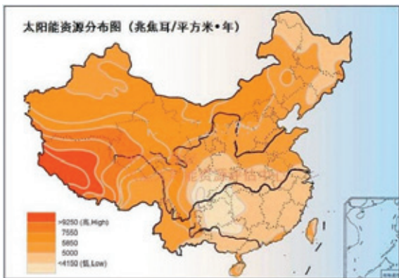
太阳能资源分布图
